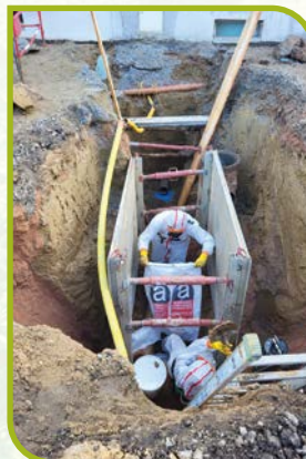
BRANCHEMENT D'ASSAINISSEMENT
